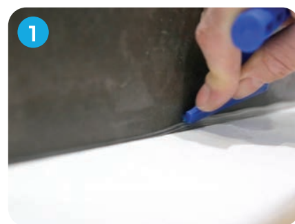
Étanchéité optimisée de la jonction Receveur/panneau décor Joint en forme de T
