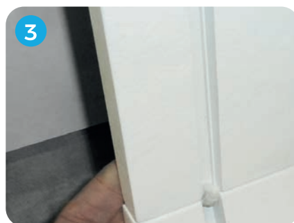
Étanchéité optimisée de la jonction Bâti-support/receveur Joint expansif de type mastic
