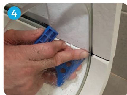
Étanchéité optimisée de la jonction Receveur/paroi en verre Joint en forme de T > Outil de montage inclus
