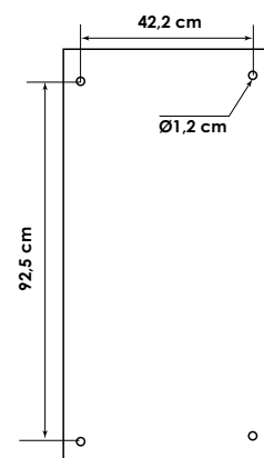
Vue arrière
